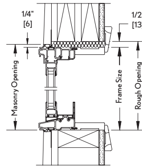
Head Jamb & Sill
