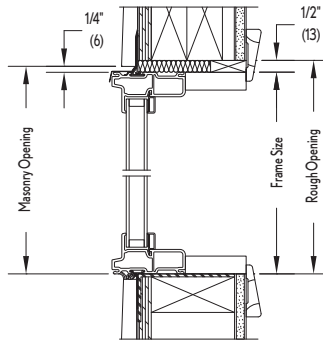
Head Jamb & Sill
